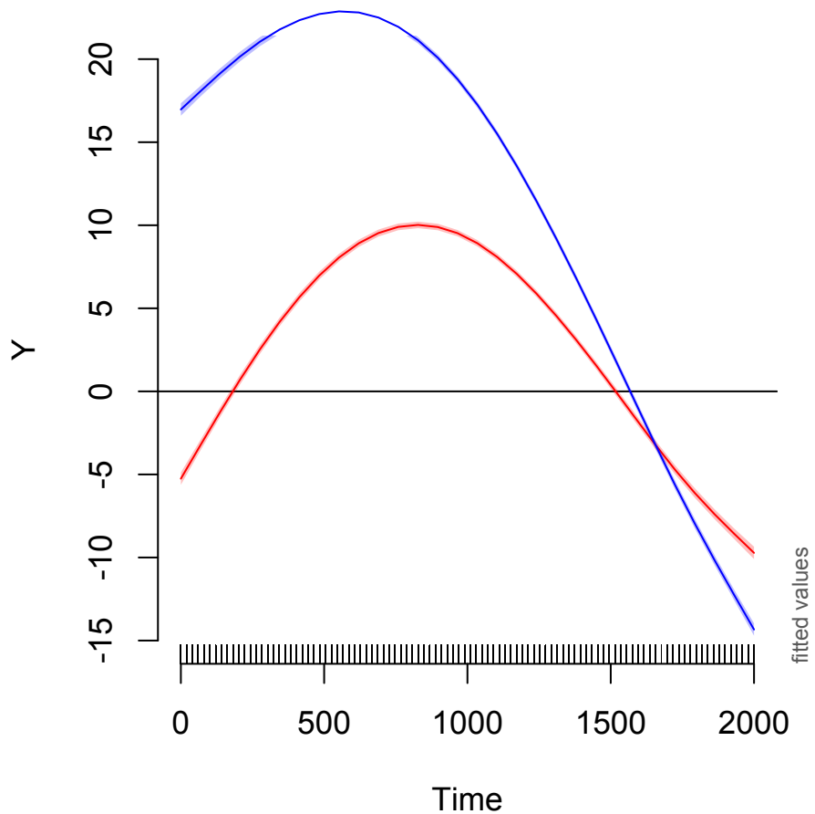
... + s(Subject) + s(Subject, Time)
