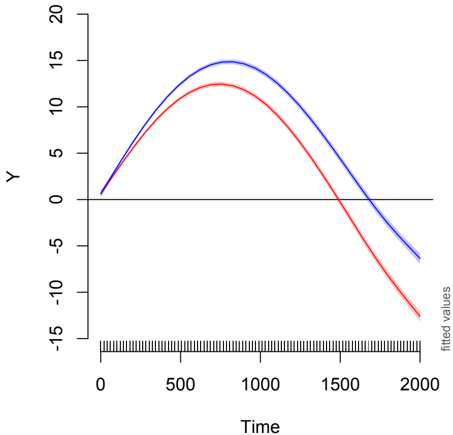
... + s(Subject)
